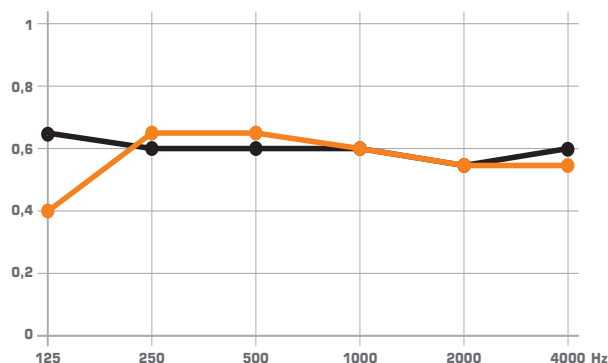
Coefficient d'absorption acoustique \alpha_p Hub'Acoustic® 29/3 (D+007)
